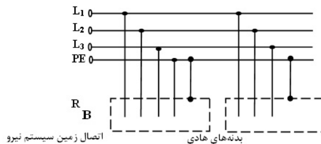
شکل پ ۲ سیستم TN-C با هادی مشترک حفاظتی- خنثی در سرتاسر سیستم.
