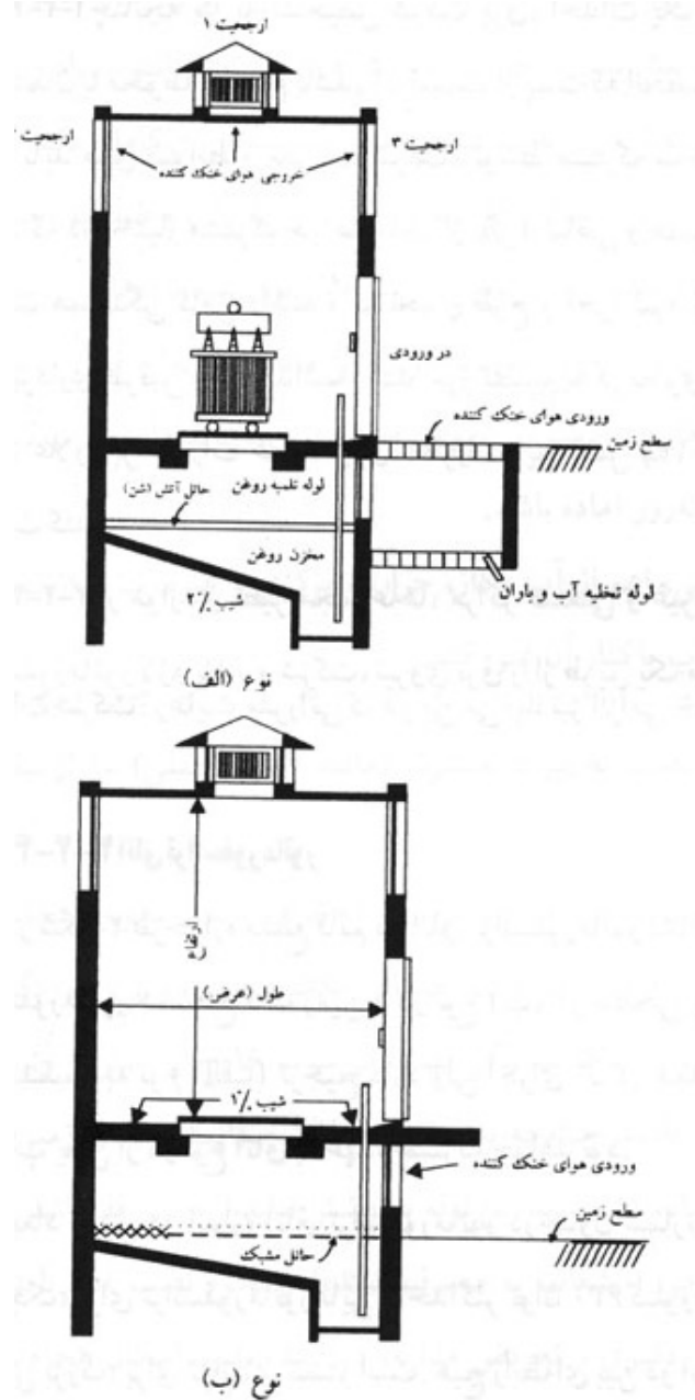
شکل ۲ طرحواره مقطع قائم دو نوع اتاق ترانسفورماتور
