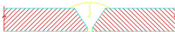
شکل ۱۷-۴-۶-۶-ت-۱ ترک در جوش
