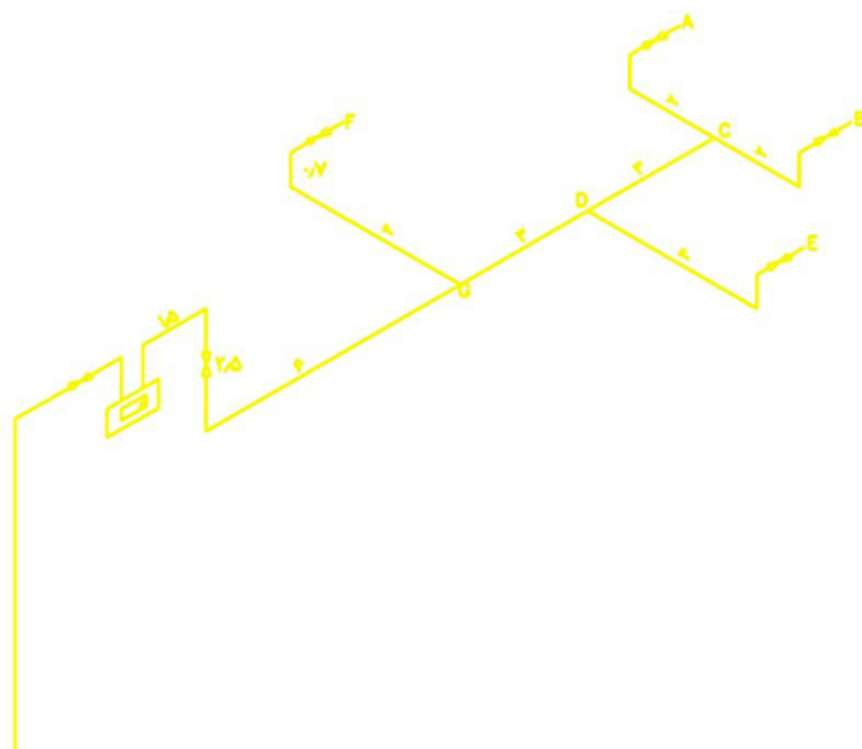
شکل پ- ۲-۱-۲ نقشه ایزومتریک
