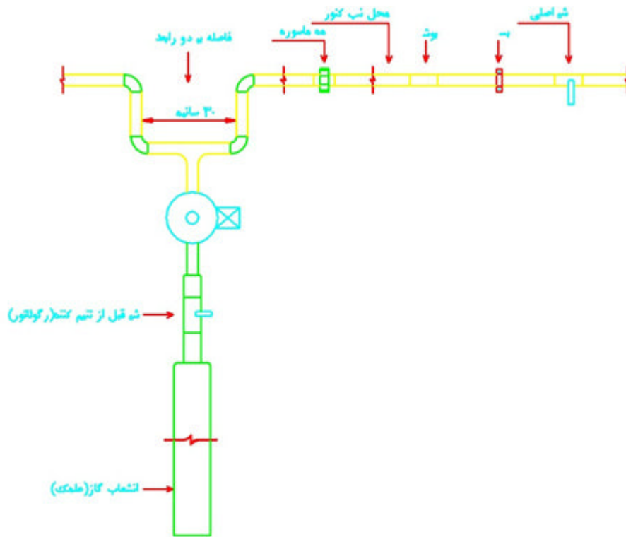
پ-۲-۲-۱ انشعاب گیری برای دو مشترک خانگی (تجاری)
