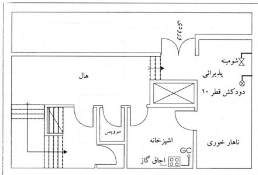
شکل پ-۱-۳-۱ نقشه لوله کشی گاز در پلان طبقه همکف
