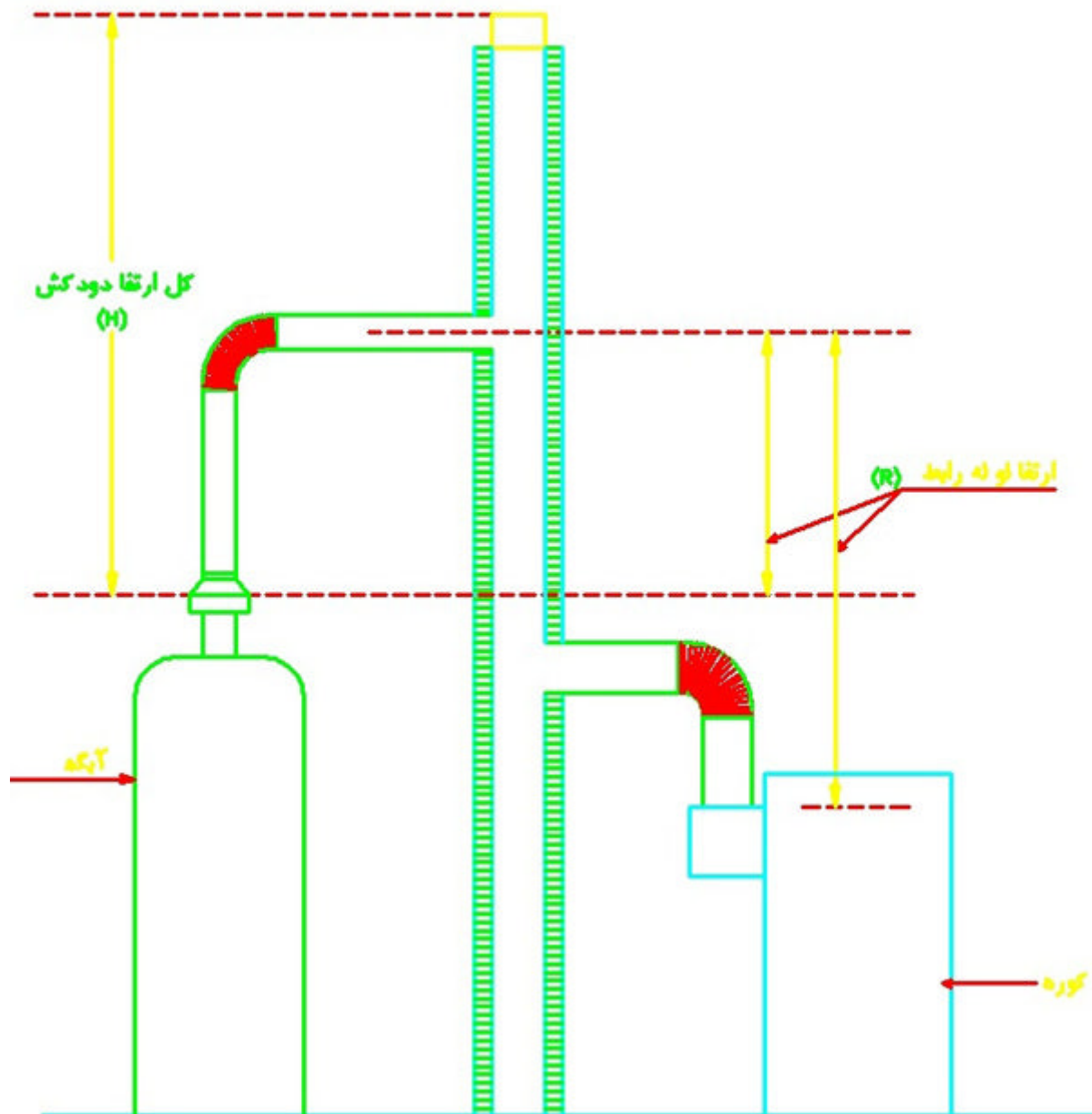
شکل ۱۷-۲-۷-۲ دودکش با مصالح ساختمانی جهت دو یا چند دستگاه گازسوز که در یک طبقه نصب شده اند.
