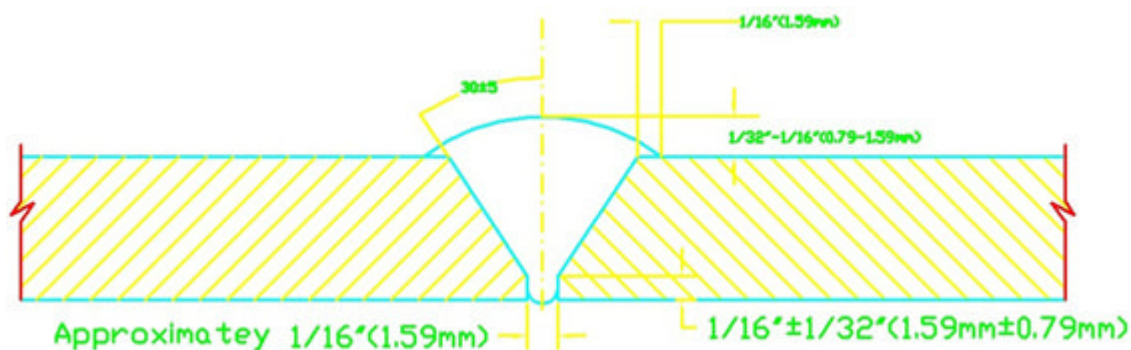
شکل ۲-۶-۴-۱۷ طرح اتصال جوش لب به لب
