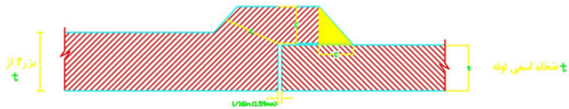
شکل ۱۷-۴-۶-۳ طرح اتصال در جوش کشویی
