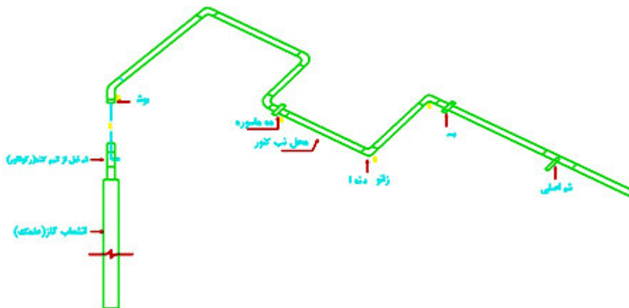
پ-۲-۲-۲ روش نصب محل کنتور گاز و لوله رابط
